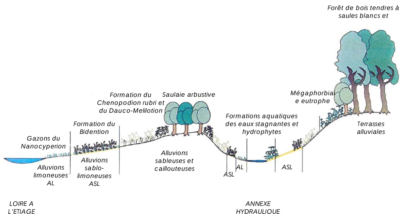
Figure n°1, schéma 1 : transect théorique des formations végétale des grèves (d'après CSNB, modifié)
