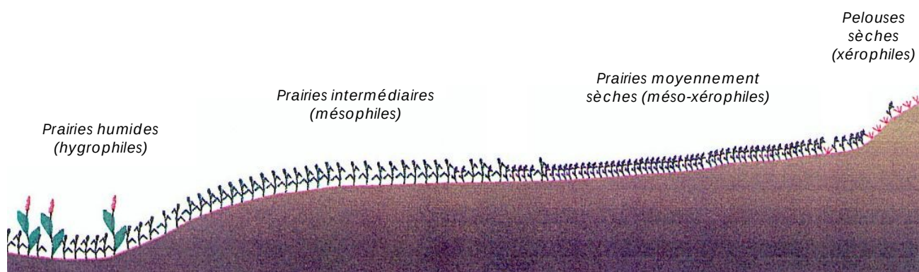
Figure n°1, schéma 3 : exemple de dynamique de colonisation d'une terrasse sableuse
