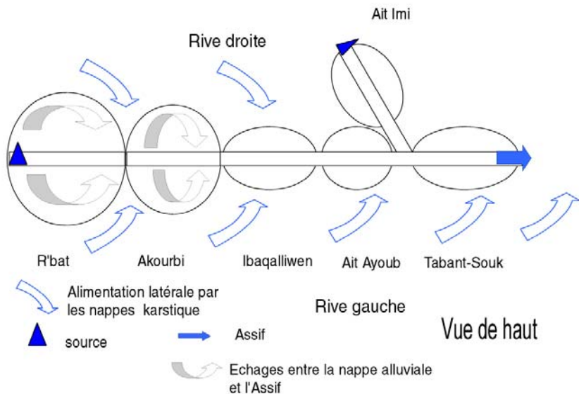
Schéma de la circulation des eaux dans l'Assif-n-R'bat
