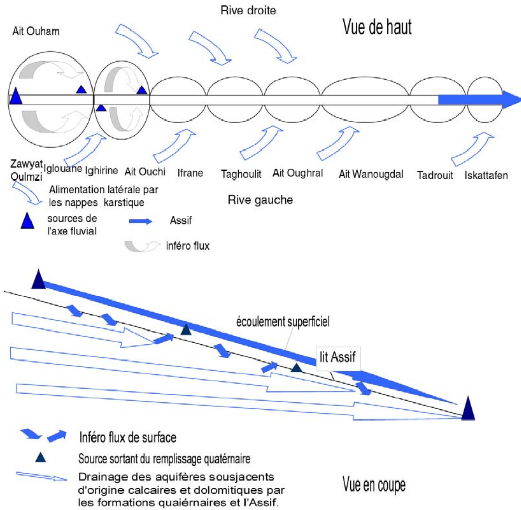
Schéma de la circulation des eaux dans l'Assif-n-Ait Hkim
