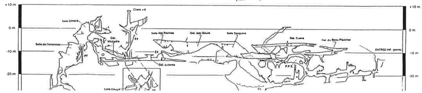
COUPES PROJÉTÉES (305° -- 125°)
